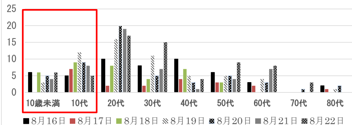
筑豊地区コロナ新規感染者年代別グラフ（人）
